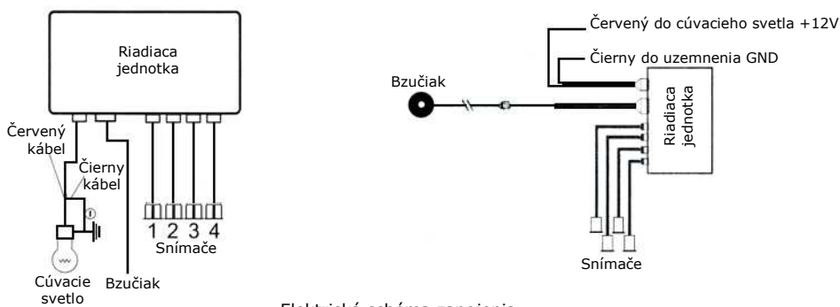
Elektrická schéma zapojenia parkovacieho snímača s bzučiakom.
